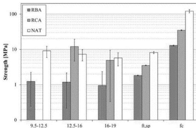
Fig. 8. Variación de la resistencia en función del tamaño de partículas de RBA, RCA y NAT (Marco et al. [44]).
