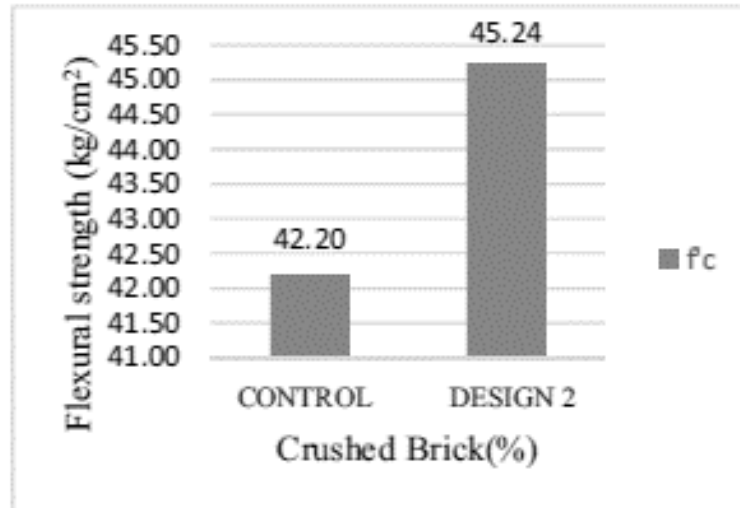
Fig. 9. Influencia del porcentaje de en la resistencia a la flexión (Fuente: Rodríguez et al. [47]).
