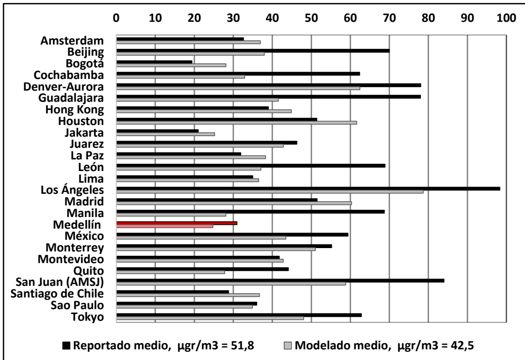
Fig. 15. Resultados reportados y modelados para el Ozono
